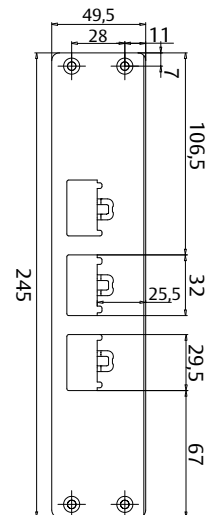
Mekaniskt slutbleck 546
