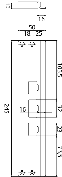
Mekaniskt slutbleck 547
